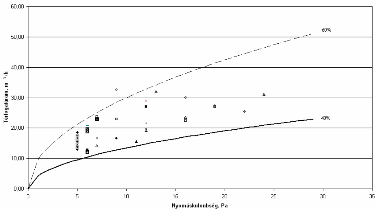
EHT-957 HU típusú, falátvezetésbe építhető légbevezetők léghozamai
