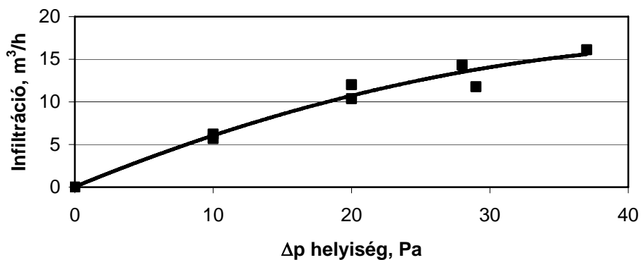
4. ábra: a tömörésvizsgálat eredménye, trendvonal és a regressziós függvény
